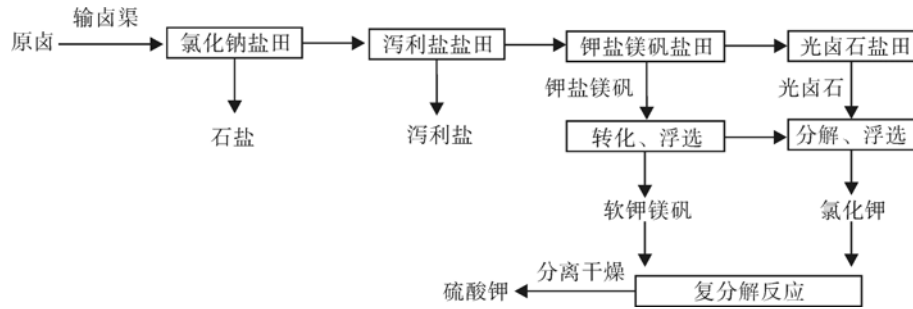
图2 罗布泊盐湖硫酸钾生产工艺流程
