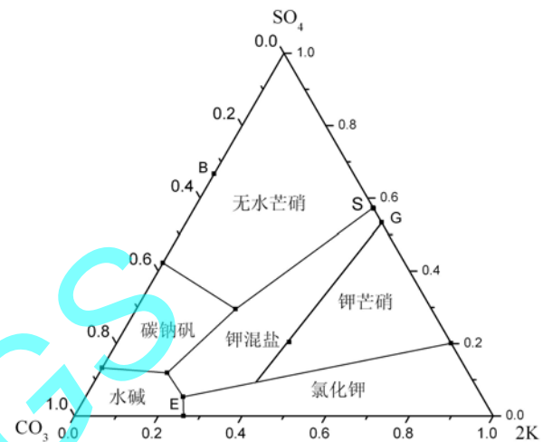
图3 \text{Na}^+ 、 \text{K}^+//\text{Cl}^- 、 \text{SO}_4^{2-} 、 \text{CO}_3^{2-} - \text{H}_2\text{O} 五元体系 25°C 介稳相图中钾混盐组成点
