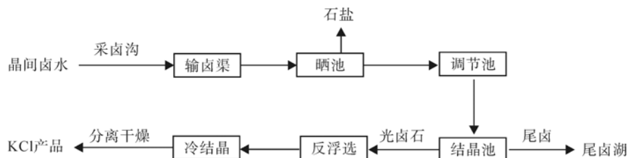
图 1 察尔汗盐湖钾肥生产工艺流程
