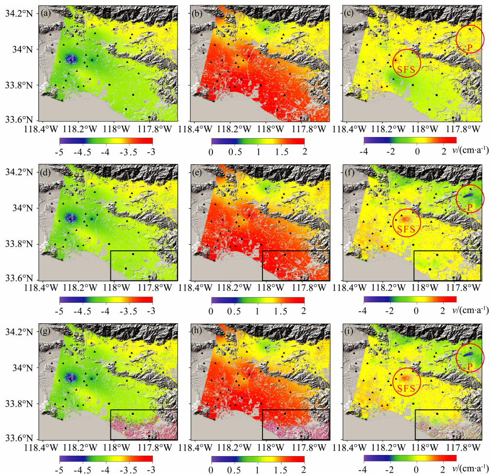
图5 (a,b,c) 南加州地区 GPS 插值得到的地表三维形变速率场;(d,e,f) BFGS 法所得的地表三维形变速率场;(g,h,i) 解析法所得的地表三维形变场 从左至右分别为东西向、南北向和垂直向结果. 黑色小三角形代表插值用的 47 个 GPS 观测站, 黑色小正方形代表验证用的 5 个 GPS 观测站. P 和 SFS 分别代表 Pomona 和 Santa Fe Springs 地区.
