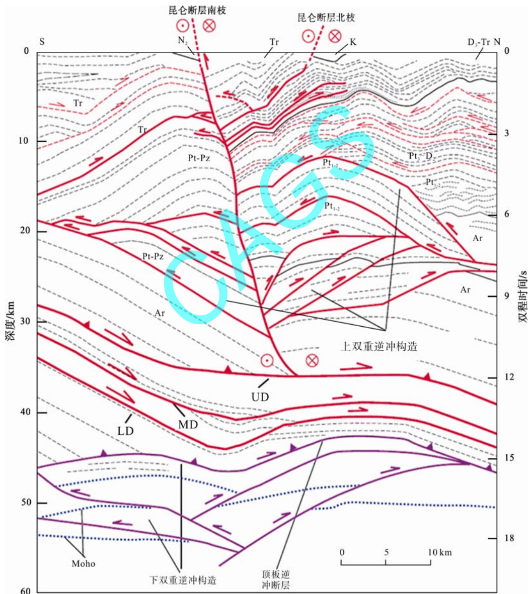
图 4 跨越昆仑左旋走滑断层的解释横剖面
