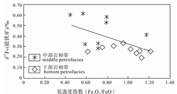
图 5 攀枝花岩体氧逸度指数与磁铁矿单矿物 Fe 同位素之间的关系图解
