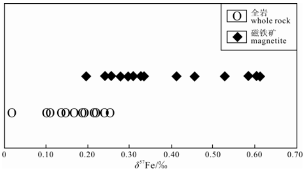
图3 攀枝花岩体朱家包包矿段样品全岩、磁铁矿 Fe 同位素分布特征
