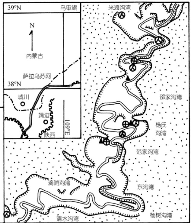
图1 萨拉乌苏遗址位置图(据董光荣等 [10] , 黄慰文等 [12] )
