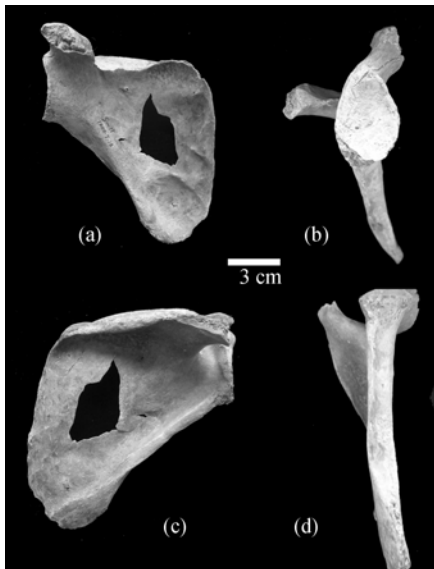
图2 萨拉乌苏遗址人类肩胛骨化石 (a)前面; (b)外侧面: 关节盂; (c)后面; (d)外侧面: 腋缘
