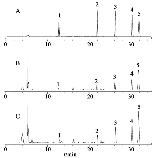
A. 对照品; B. 80 °C 烘干样品; C. 乳制样品; 1. 日蟾毒它灵; 2. 蟾毒它灵; 3. 蟾毒灵; 4. 华蟾酥毒基; 5. 酯蟾毒配基
