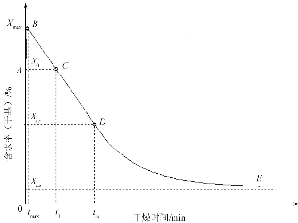
注： X_0 、 X_{max} 、 X_{cr} 和 X_{eq} 分别为物料原始干基含水率、蒸汽凝结结束时物料的干基含水率、临界干基含水率和平衡含水率，%； t_{max} 、 t_1 和 t_{cr} 为蒸汽凝结结束时对应的干燥时间、物料干燥过程中其干基含水率等于初始含水率时对应的干燥时间、物料含水率降低到临界干基含水率所对应的干燥时间，min。
