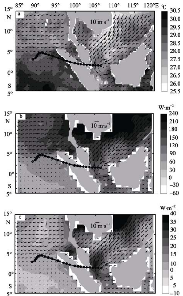
图 2 台风“画眉”生成前 5 天的平均 SST (a)、潜热(b)、感热(c)与风场(箭头)的合成图 图中黑色圆点连线表示台风路径 Fig. 2 Synthesis map of average SST (a), latent heat (b), sensible heat (c) and wind field (arrows) of 5 days before Typhoon Vamei was generated
