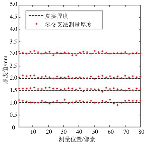
图6 聚乙烯板模型厚度测量结果
