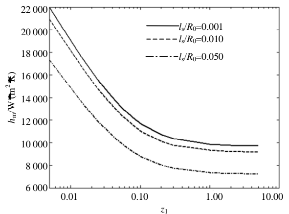
图4 平均换热系数受速度滑移系数的影响曲线
