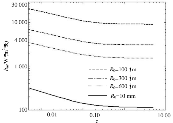
图3 平均对流换热系数受尺寸效应的影响曲线
