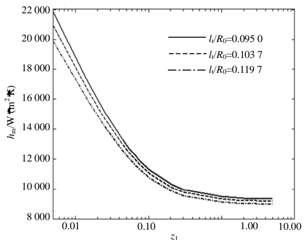
图5 平均换热系数受温度跳跃系数的影响曲线
