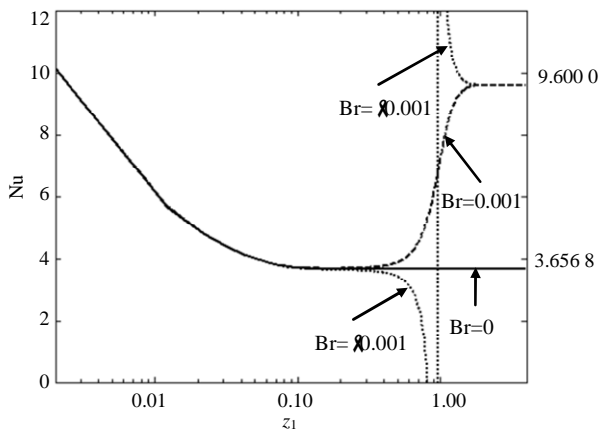
图2 Br数对努塞尔数的影响
