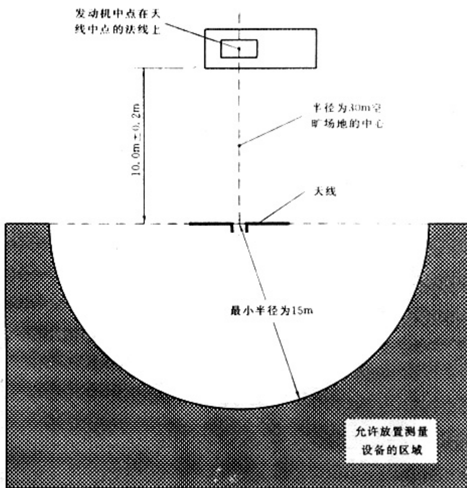
图 4 测量场地
