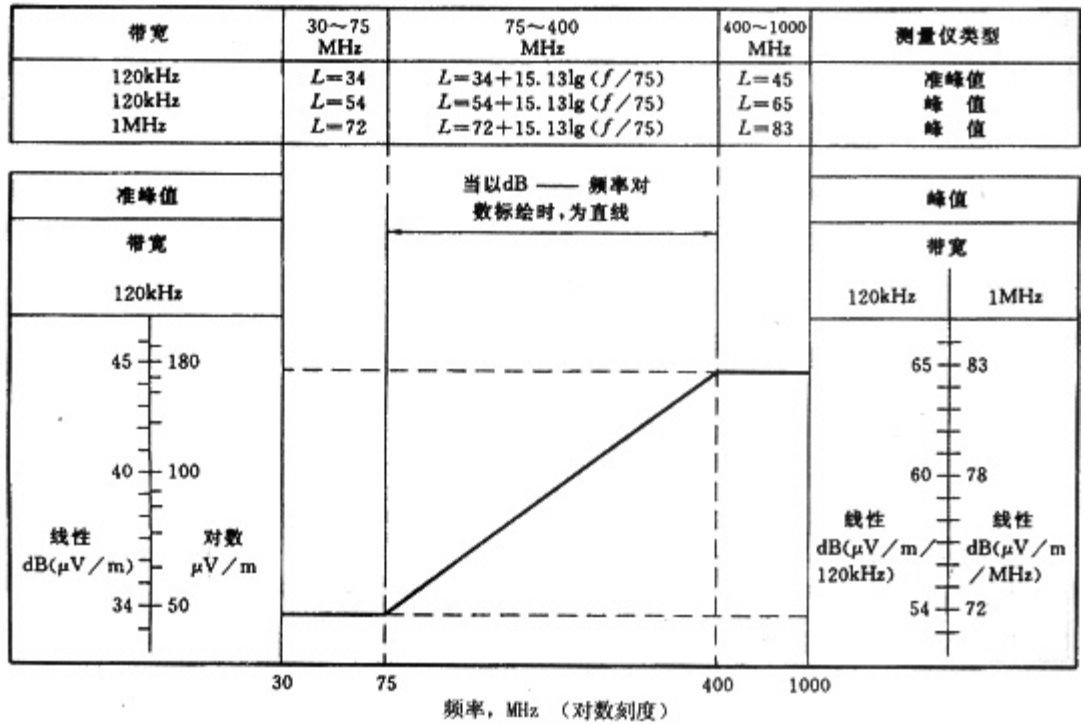
骚扰限值 L (dB( \mu V/m)) (在频率为 f MHz时)
