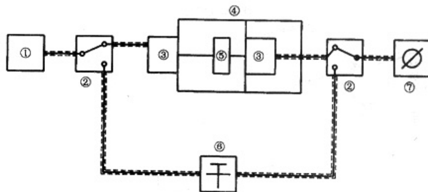
①—信号发生器；②—同轴开关；③—固定衰减器(10dB)；④—试验箱； ⑤—受试样品；⑥—校准的可变衰减器；⑦—测量仪器 注：①、②、③、⑥和⑦均须具有相同的特性阻抗。
