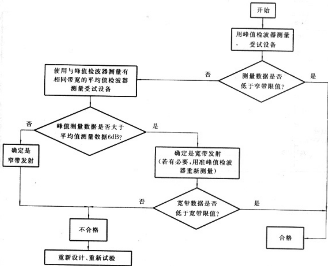
图1 确定辐射骚扰合格与否的流程图
