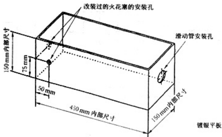
图 E4 试验箱详图
