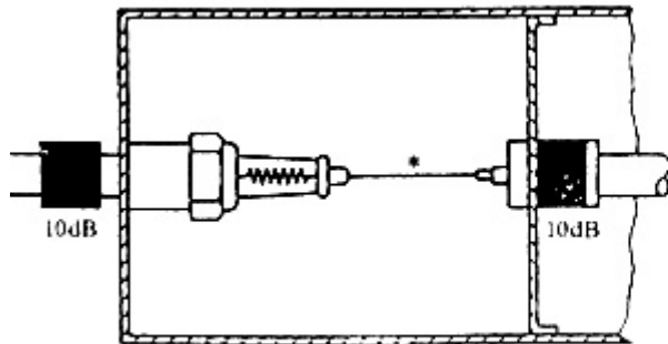
图 E7 噪声抑制火花塞
