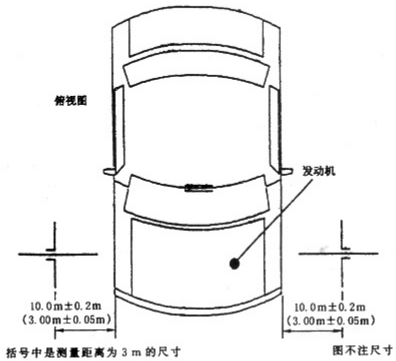
图 6 测量辐射骚扰的天线位置——水平极化
