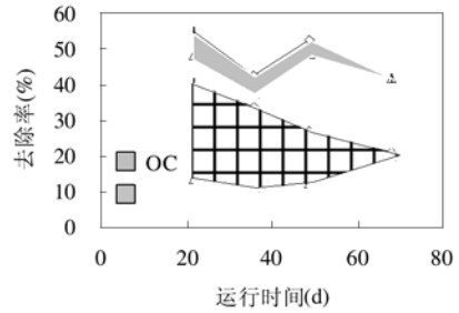
图 5 PAC-MBR 与块状填料-MBR 有机物去除率差异随时间的变化
