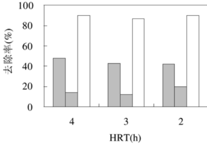
图 4 不同 HRT 块状填料-MBR 的污染物去除效果 Fig.4 Pollutant removals of MBR filled with nubby carriers under different HRTs
