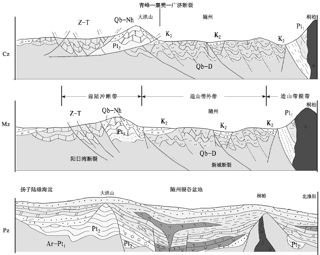
图 3 东秦岭造山带南缘构造演化模式
