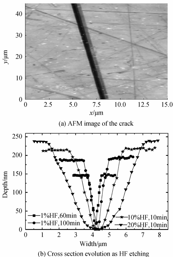
图 3 划痕原子力形貌及其剖面结构随刻蚀时间、HF 浓度的变化
