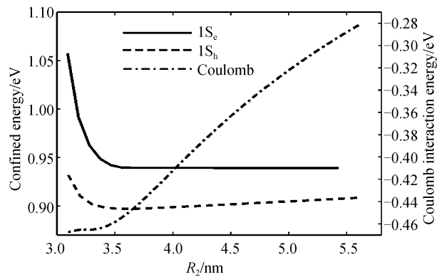
图 8 在内半径 R_1=3 nm 保持不变时, 载流子的能量及相互库仑作用能随外半径 R_2 增大的变化
