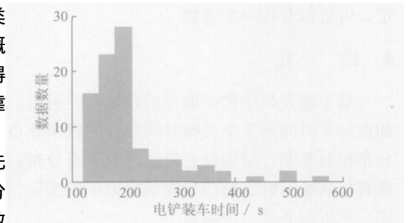
图 2 电铲装车时间的直方图
