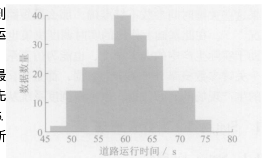
图 1 道路运行时间的直方图
