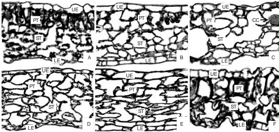
图1 不同锰浓度处理对垂序商陆叶片形态结构的影响
