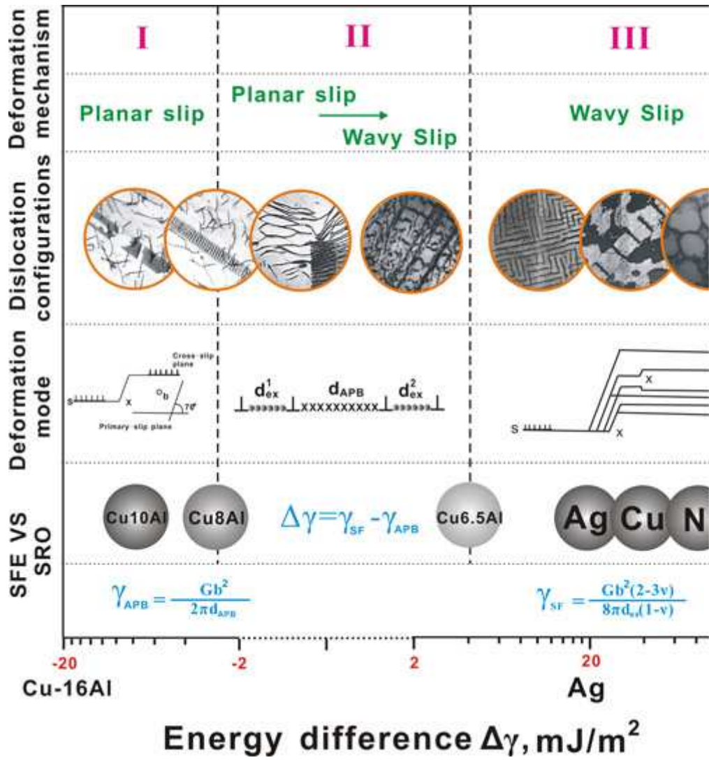
图2 面心立方金属或合金循环变形过程中不同位错组态形成的基本判据——层错能与短程有序的影响。
