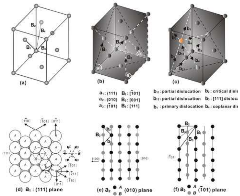
图1 不同取向晶体位错组态的形成原因一位错运动与滑移系选择：(a) 潜在柏氏矢量；(b) 滑移与剪切系统；(c) 位错组态的运动；(d)，(e)，(f) 滑移与剪切系统的选择。
