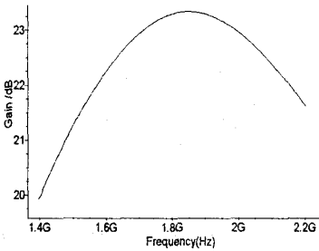
图6 LNA的正向增益
