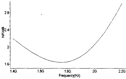
图5 噪声系数NF仿真结果
