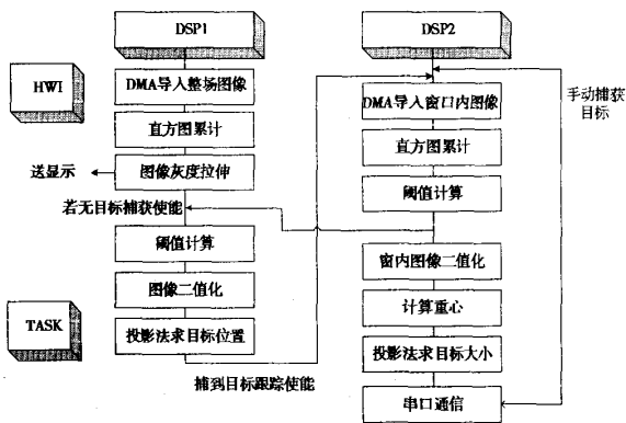
图 3 电视跟踪程序原理框图
