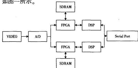
图 1 电视跟踪系统硬件框图
