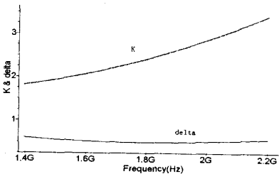
图7 LNA的稳定因子
