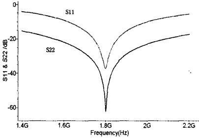
图4 LNA的S11和S22模拟结果
