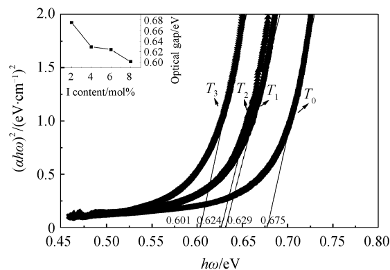
图 5 玻璃样品 (\alpha h\omega)^2 和 h\omega 的关系(插图为直接带隙 E_{\text{opt}} 与 I 含量的关系)
