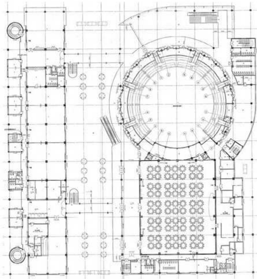
二层平面
