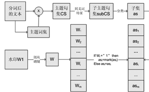
图2 水印嵌入算法流程
