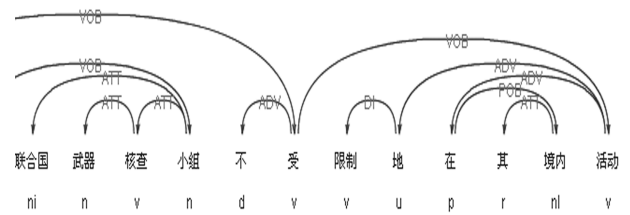
图3 依存句法分析截图
