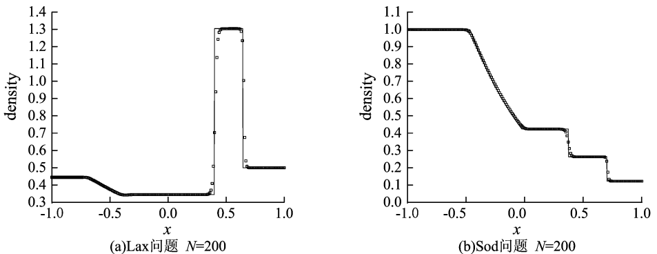
图 2 Euler 方程的 Riemann 初值问题
