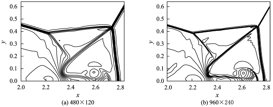
图 7 双马赫反射问题的密度从 1.5 到 22.7 的 30 条等值线局部放大图
