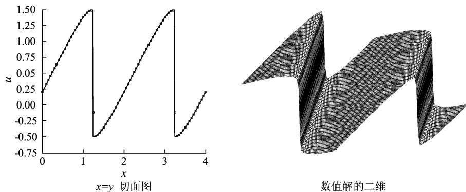
图 5 二维 Burgers 方程, 80 × 80
