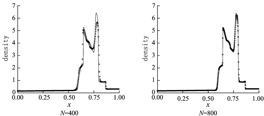
图 4 Euler 方程强激波碰撞问题
