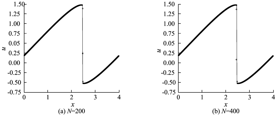
图 1 一维线性标量 Burgers 方程
