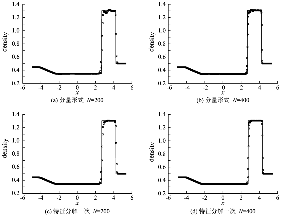
图 8 Lax 激波管问题
