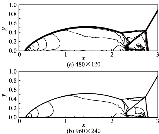
图 6 双马赫反射问题的密度从 1.5 到 22.7 的 30 条等值线图
