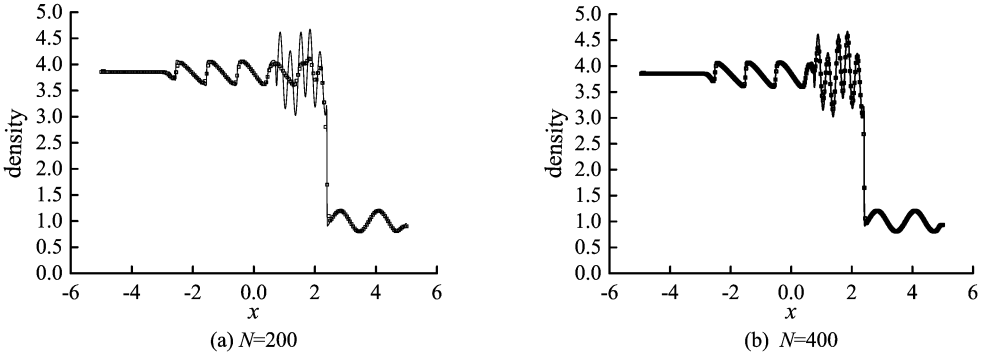
图 3 Euler 方程激波密度波碰撞问题
