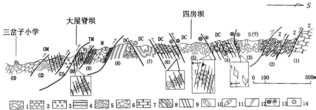
图 2 略阳县三岔子地质构造剖面
