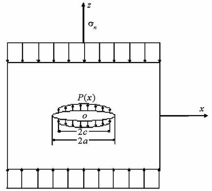
图2 CO 2 封存于砂岩透镜体中的币形裂纹计算模型
