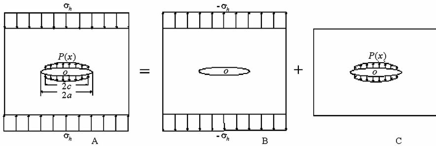
图3 计算币形裂纹模型应力强度因子的叠加原理
