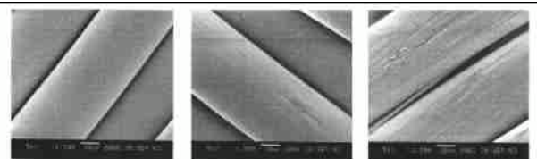
(a) 未经处理的PP纤维 (b) 氧气处理后的PP纤维 (c) 氧气处理后的PP纤维 条件: 100W, 30 mL/min, 30s 条件: 300W, 30 mL/min, 180s
