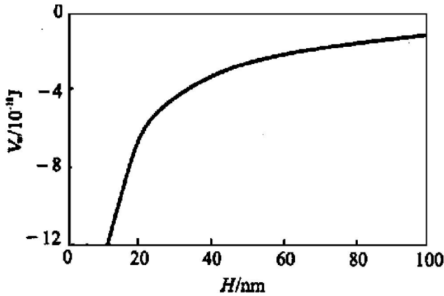
图 1 一水硬铝石与含硅脉石矿物间的范德华相互作用能 Fig. 1 Van Der Waals interaction between diaspore and silicate minerals
