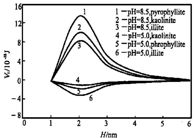
图 2 一水硬铝石与含硅脉石矿物间的静电相互作用能
