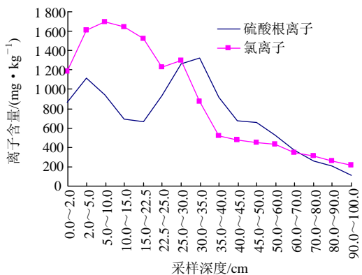
图 8 岩体内氯离子和硫酸根离子含量随深度变化曲线
