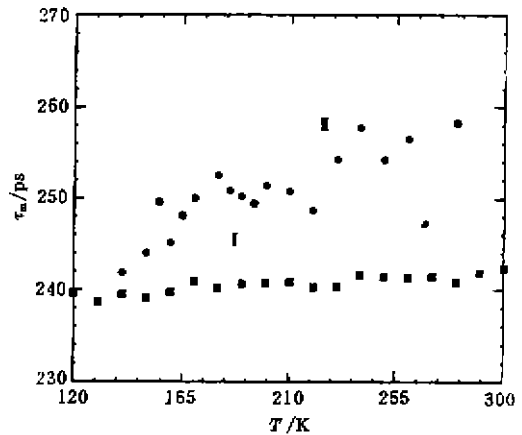
图 2 500 MeV Ne 辐照前后 InP 中正电子平均寿命随温度的变化 I 辐照前的变化情况, II 在 10^{14} ions/cm 2 剂量辐照后的变化情况.
