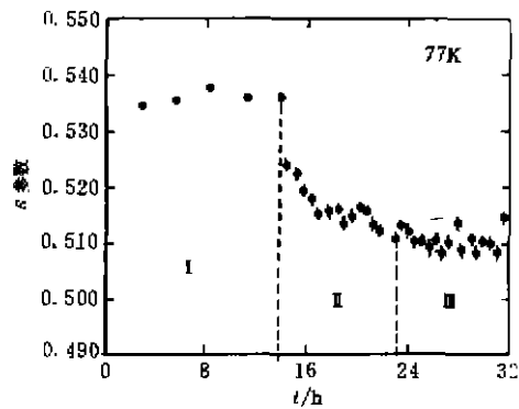
图 4 500 MeV Ne 辐照 InP 时 S 参数随时间的变化
