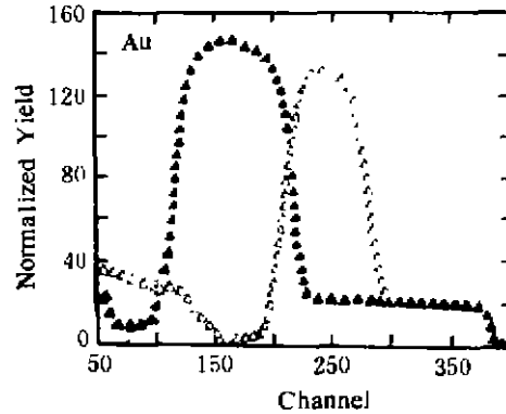
图 3 在液氮温度下,用 500 MeV I 离子辐照三明治结构(非晶态 \text{Ni}_3\text{B} -Au-非晶态 \text{Ni}_3\text{B} )到 3 \times 10^{15} 离子/ \text{cm}^2 时记录到的 RBS 谱.实心三角代表辐照样品,空心三角代表未辐照样品
