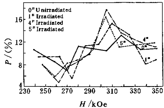
图 2 铁磁相超精细场的几率分布
