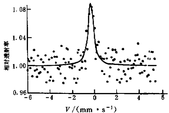
图 4 在 77K 温度下 57 Fe 注入 Cu 的穆斯堡尔谱
