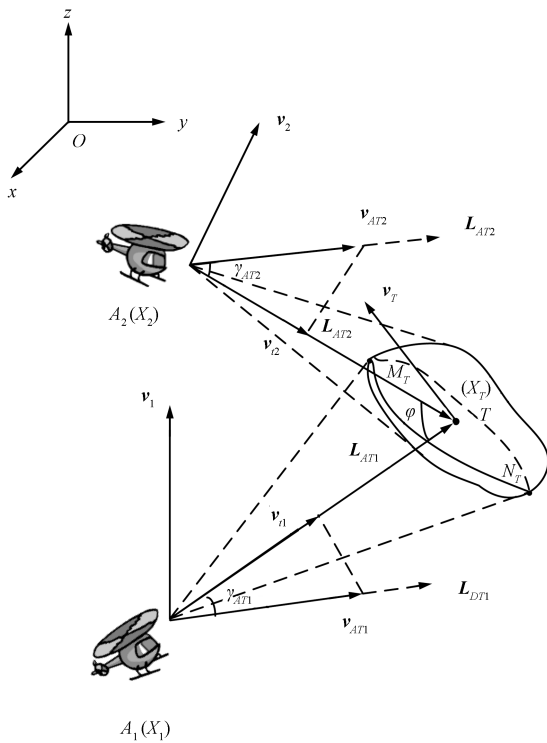
图 5 相对速度空间下目标追踪原理 Fig. 5 Target tracking in RVCs
