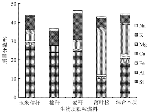
图2 中国生物质颗粒燃料灰渣中化学成分含量
