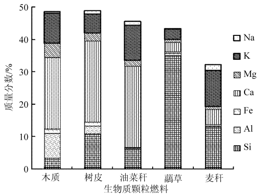
图1 瑞典生物质颗粒燃料灰渣中化学成分含量
