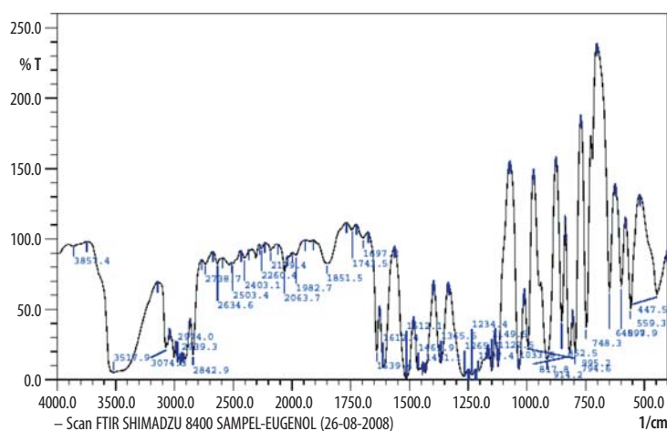
Fig. 10. IR spectra of eugenol
