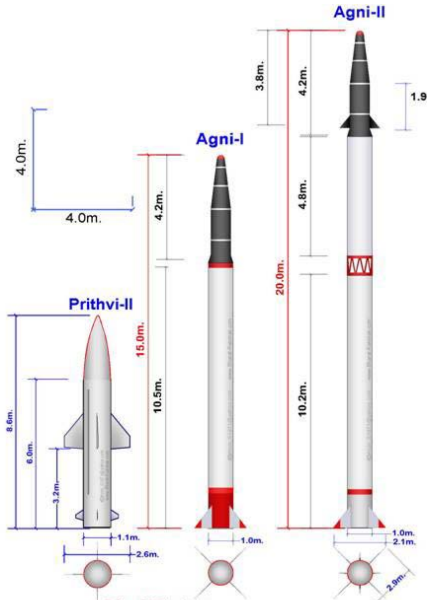
印度展示普里特维地对地导弹同“烈火”1型、2型的比较 [资料图片]
