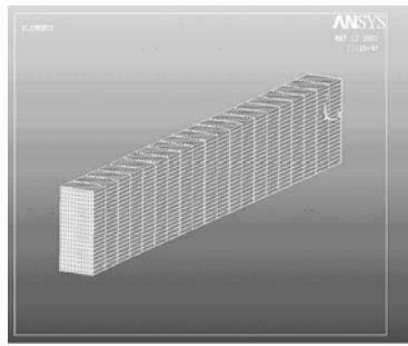
图2 柱混凝土网格(20×10×20)
