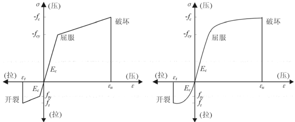
(a)线弹性—线性硬化塑性—断裂 (b)线弹性—非线性硬化塑性—断裂
