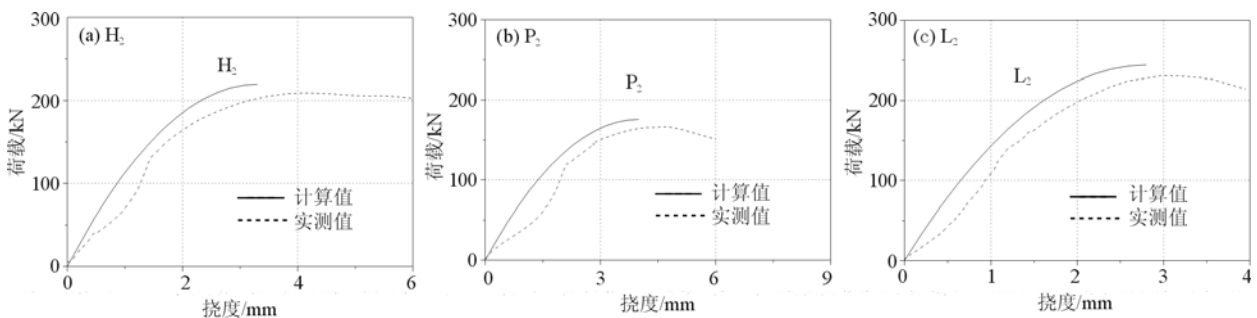
图7 偏心柱 e_0=0.2h 荷载—挠度关系曲线
