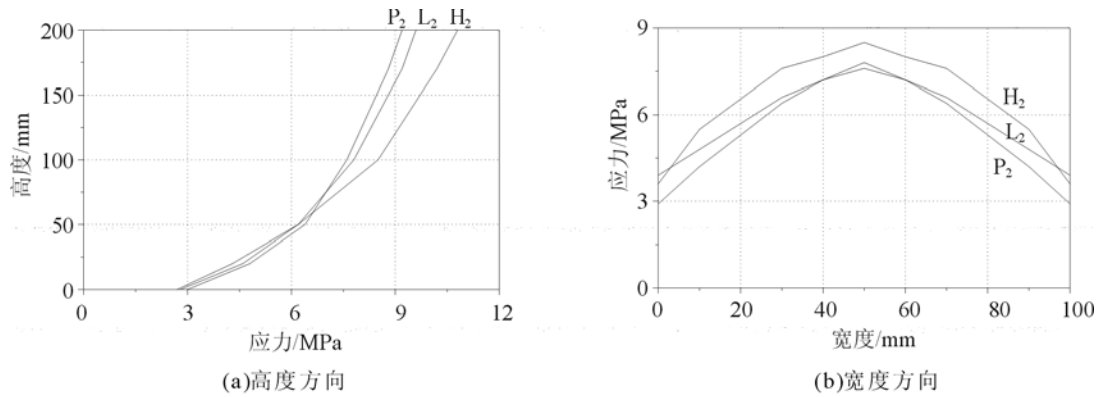
图5 偏心受压 e_0=0.2h 应力分布曲线
