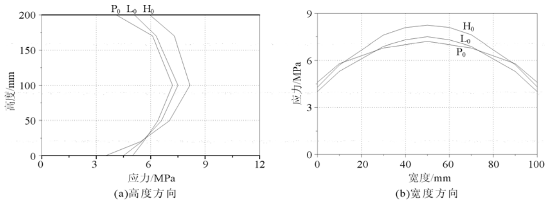
图4 轴心受压柱形心轴上应力分布曲线
