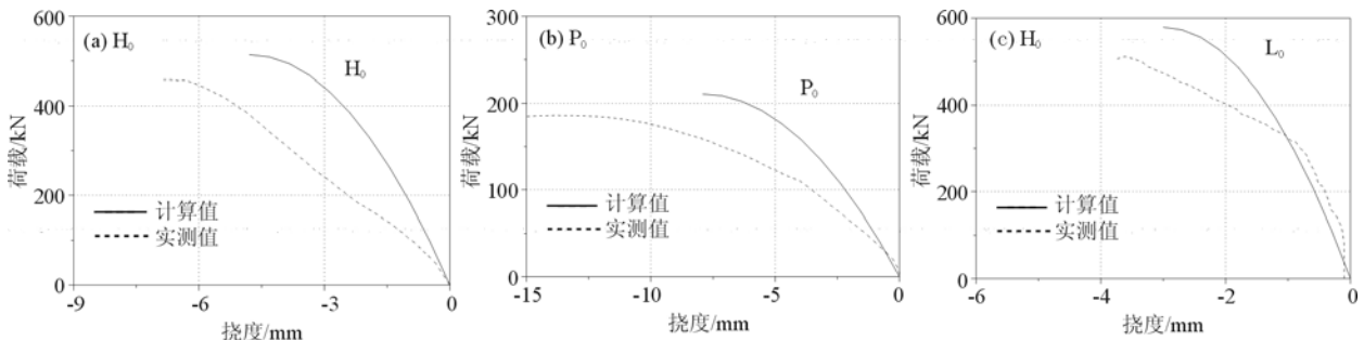
图6 轴压柱荷载挠度关系曲线
