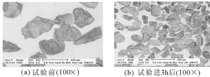
图7 试验不同阶段的石英砂形貌
