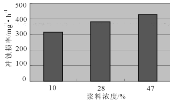
图5 冲蚀磨损率随浆料浓度的变化
