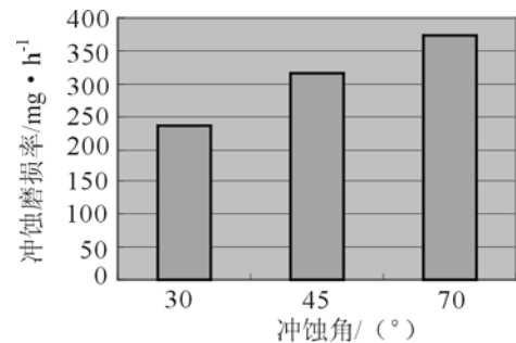
图4 冲蚀磨损率随冲蚀角的变化
