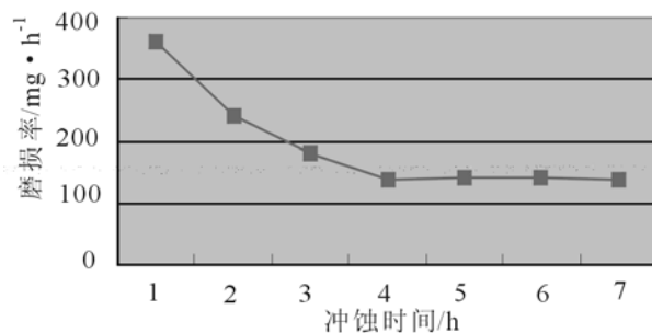
图6 磨损率随冲蚀时间的变化
