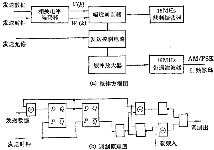
图 4 AM/PSK 调制器
