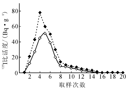
图 3 土壤淋溶液中碘含量的动态变化 ◇——青紫泥; ◆——小粉土
