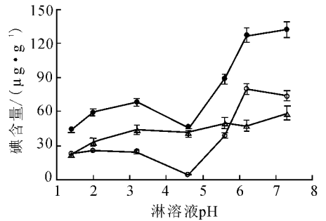
图 4 土壤淋溶液中碘含量随pH的变化 ●——总碘; ▲—— \text{I}^- ; ○—— \text{IO}_3^-
