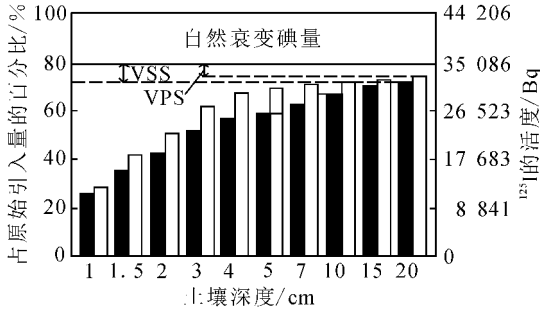
图 2 土壤中 ^{125}\text{I} 随深度的累计分布与 ^{125}\text{I} 的丢失分配图 □——青紫泥; ■——小粉土; VSS——小粉土中 ^{125}\text{I} 的挥发量; VPS——青紫泥中 ^{125}\text{I} 的挥发量;
