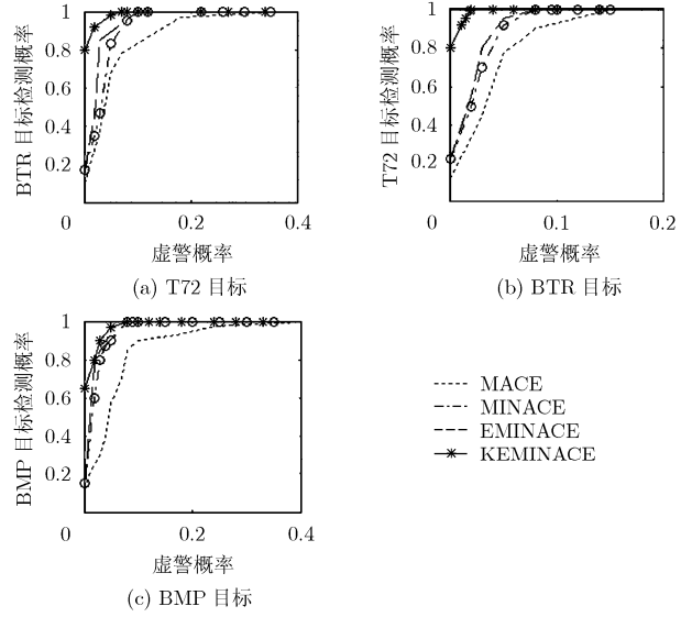
图2 ROC曲线
