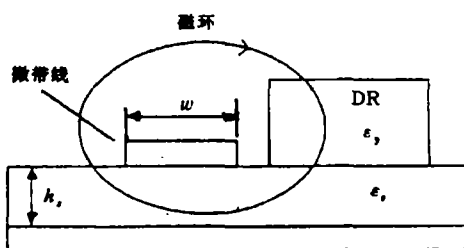
图 3 微带线激励的回音壁模
