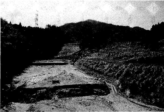
第6図 麻生溜池の堤体崩壊と土砂流出の状況 (1997年7月31日撮影).
