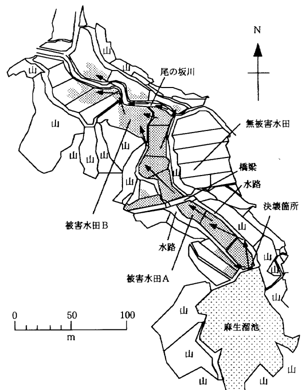
第5図 麻生溜池および堤体の決壊により埋没した水田の範囲と氾濫水の広がりの状況。
