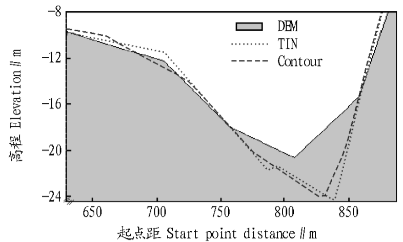
图3 栅格DEM、TIN、等高线获取断面高程数据
