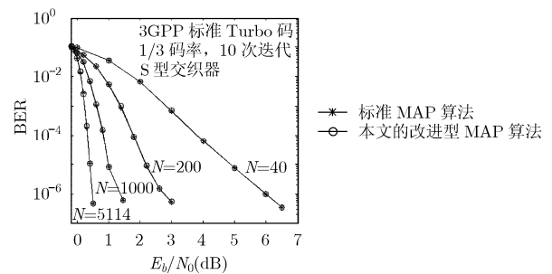
图 2 改进型 MAP 算法的纠错性能
