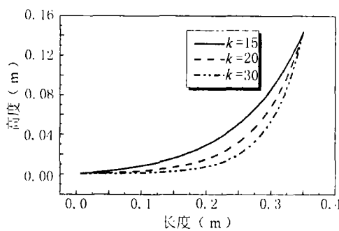
图 5 天线指数渐变曲边
