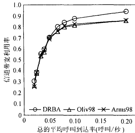
图 5 小区内的信道带宽利用率
