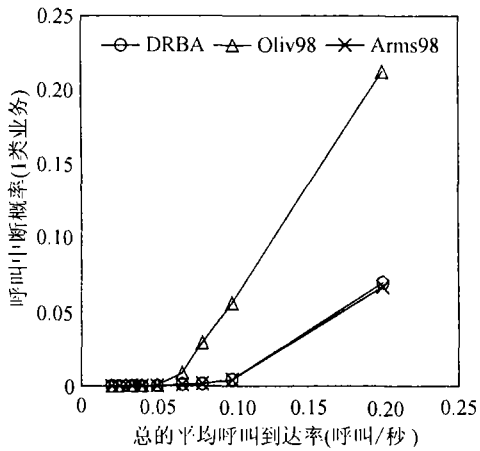
图 1 1类业务的呼叫中断概率 (CDP)
