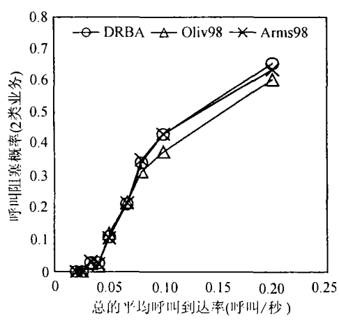
图 4 2类业务的呼叫阻塞概率 (CBP)
