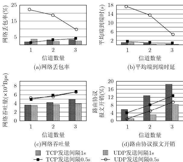
图3 TCP 和 UDP 协议对 AODV-LFA 性能的影响
