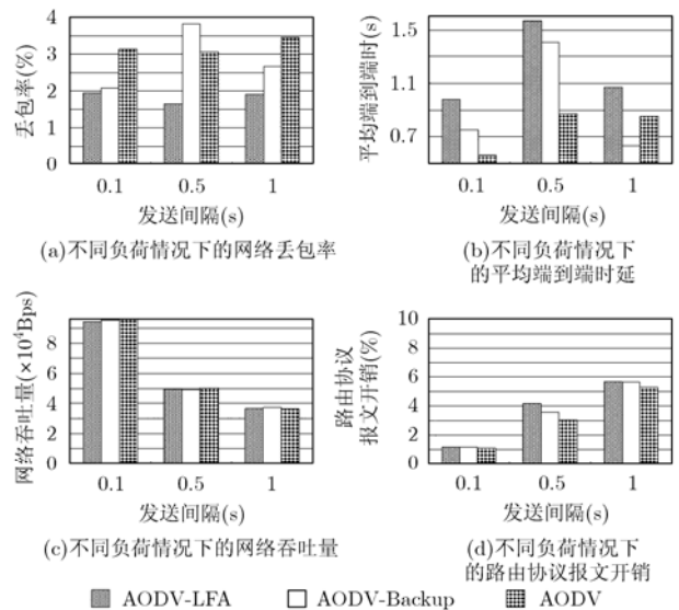
图 2 不同负荷情况下的 AODV, AODV-Backup 和 AODV-LFA 性能比较
