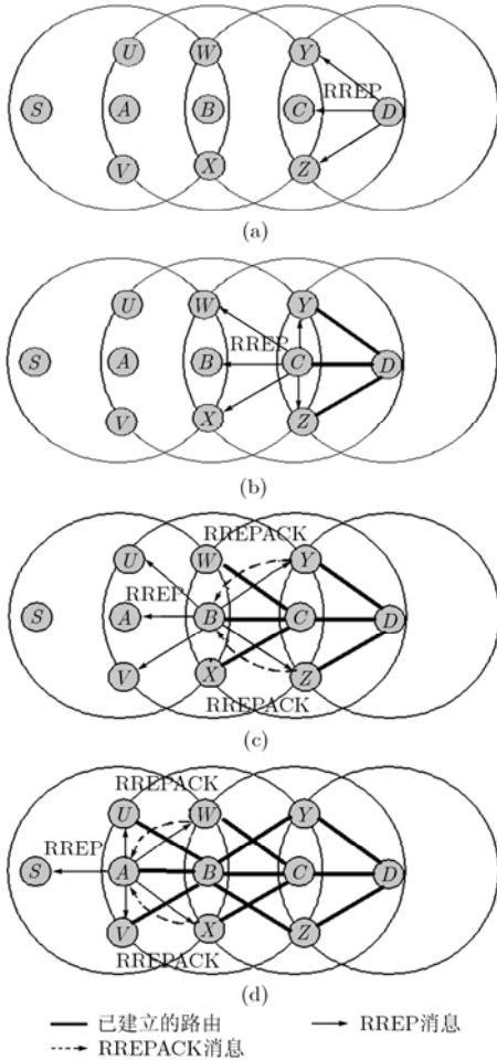
图 1 AODV-LFA 重路由路径建立示例
