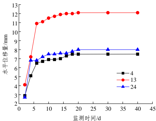
图 7 坡顶位移典型曲线
