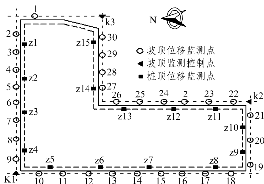
图 6 位移监测点布置
