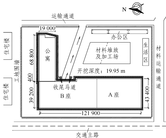
图1 基坑平面图(单位: mm)
