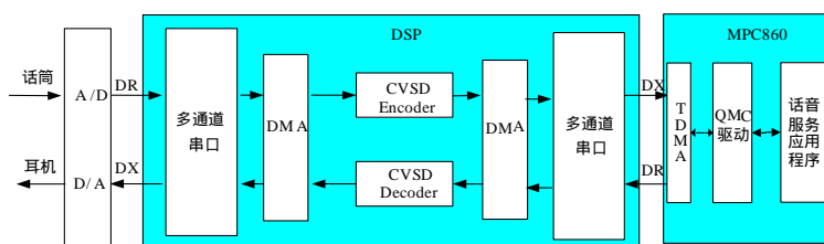
图 1 系统构架
