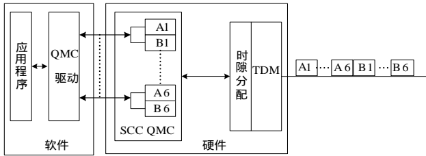
图 2 QMC 接口
