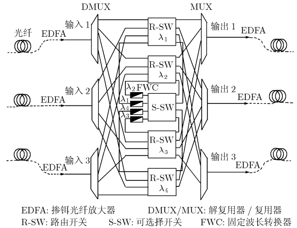
图1 全光波长路由器结构
